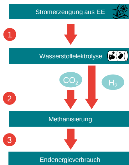
Abbildung 25 Synthetisches Methan
